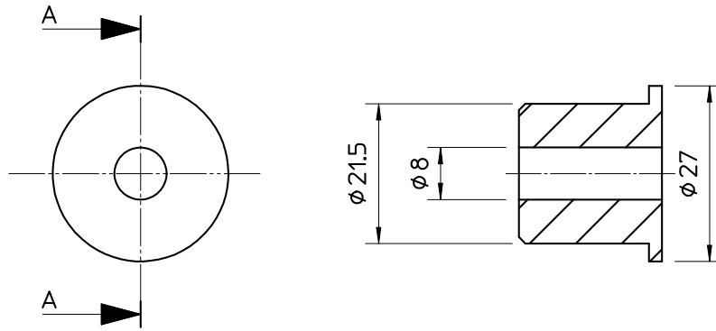
DOORSNEDE A-A
